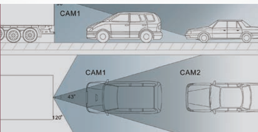
DBC 114066 TS / DBC 114047 TW Sichtfeld für Twin- und Tiltkameras Example for Viewing field of Twin- and Tiltcameras
